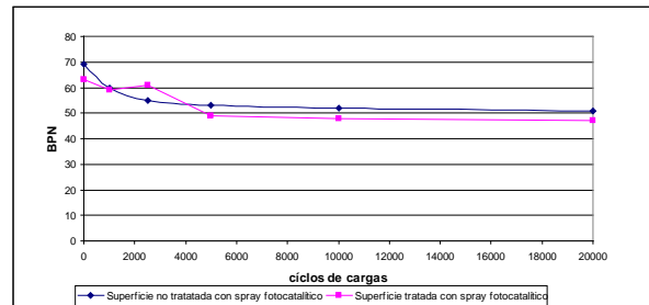
Figura 13. Ensayo de resistencia al deslizamiento aplicado sobre las superficies de rodadura tratadas y sin tratar.
