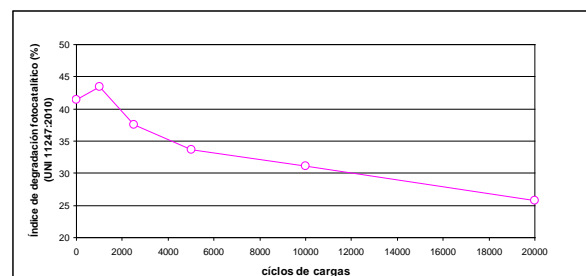
Figura 14. Curva de análisis de la resistencia al deslizamiento y eficiencia fotocatalítica de testigos extraídos de rodadura de tramo urbano.
