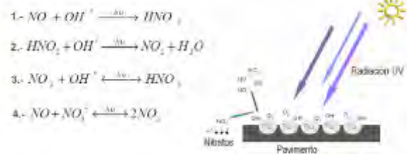
Figura 1. Mecanismo de Reacción y Degradación de los óxidos de nitrógeno en presencia del fotocatalizador \text{TiO}_2 .
